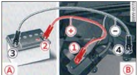
איור 353 התנעת הרכב בעזרת מצבר של רכב אחר (A) - מספק, ששמל, (B) - פרוק
